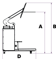
Emballasjepresse Orwak Flex 1100 MÅL mm
