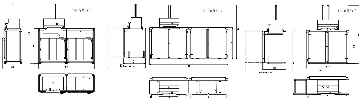
Bilde av en-kammer modell for 660 liter beholdere.
